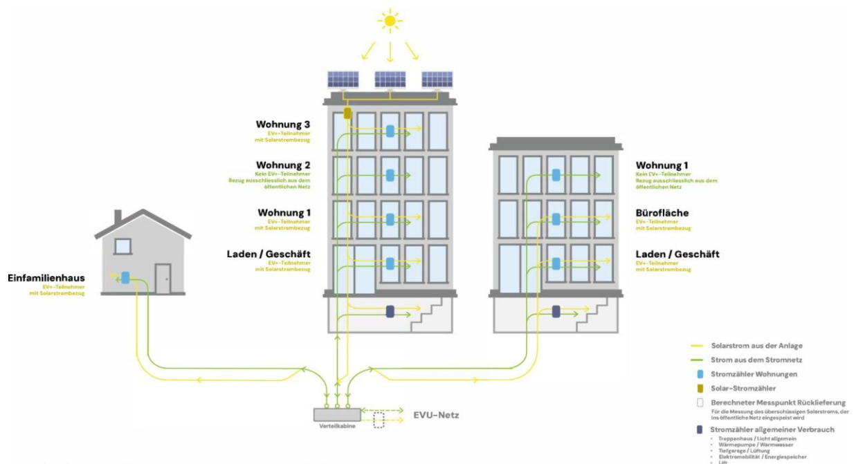
Grafische Darstellung EV PLUS mit mehreren Gebäude
