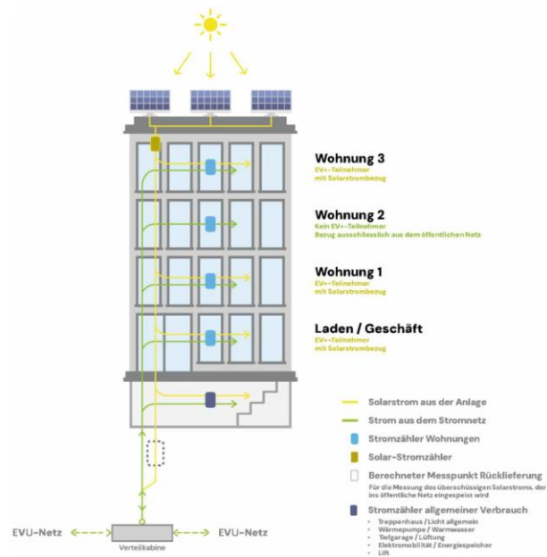
Grafische Darstellung EV PLUS mit einem Gebäude
